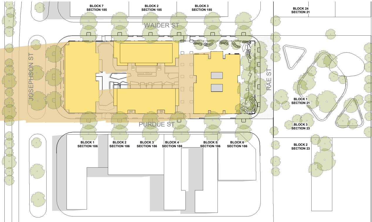
SHADOW DIAGRAM - EQUINOX - 9AM
